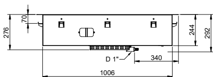
Zadní strana
